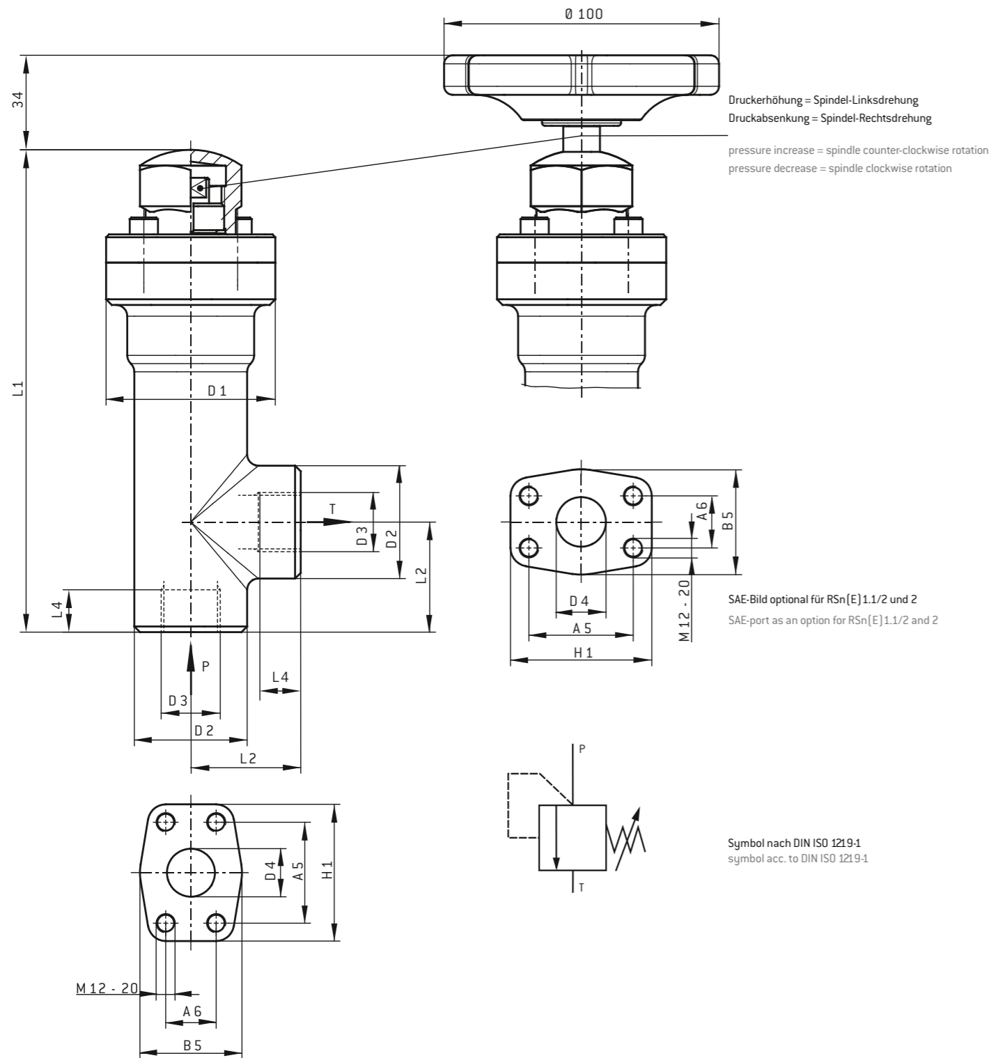
Abb. 2: Maßzeichnung
