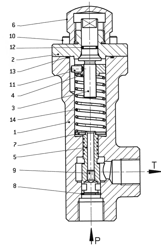
Abb. 1: Schnittbild
