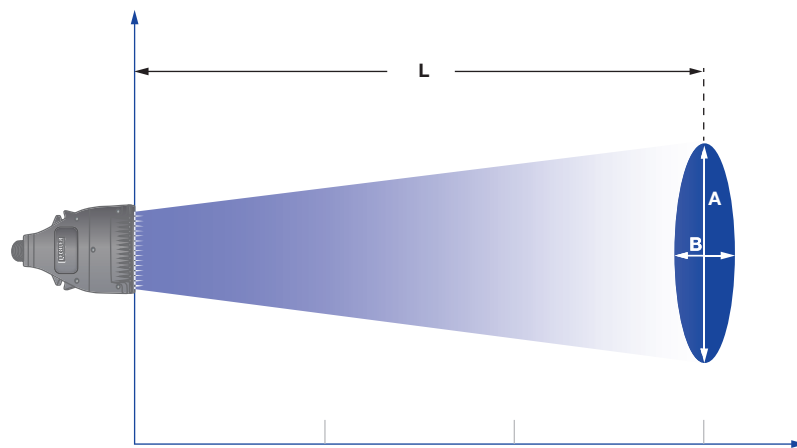
Strahlausbreitung der Baureihe 600.606
