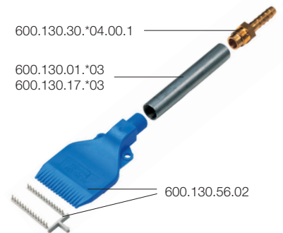
600.130.56.01 mit Zubehör *01 = 1.0711 / 17 = AISI 316Ti / 30 = Messing
