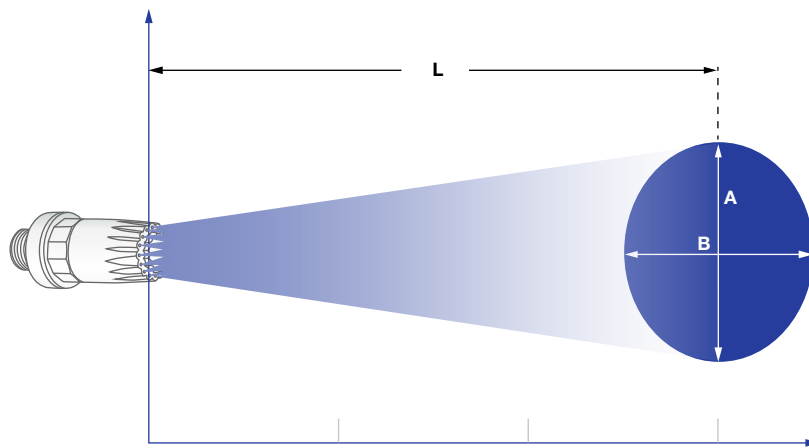
Strahlbreitung der Baureihe 600.326.5K
