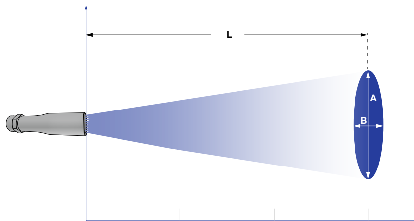
Strahlausbreitung der Baureihe 600.382.35.AE
