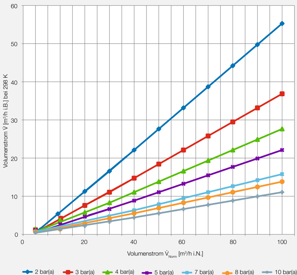
Abbildung 1: Zusammenhang zwischen Norm- und Betriebsvolumenstrom
