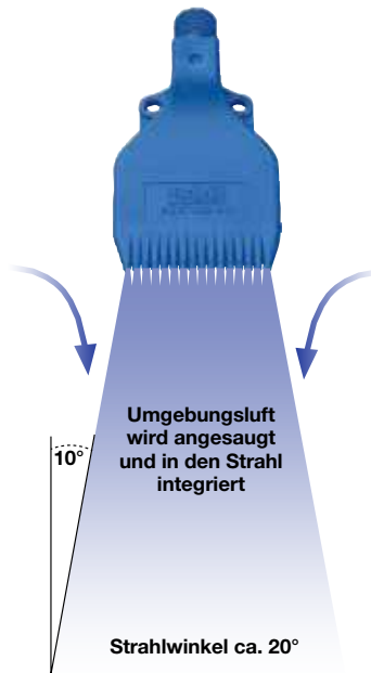
Abbildung 2: Strahlaufweitung einer Druckluftdüse
