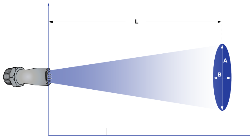
Strahlbreitung der Baureihe 600.386.01.AE
