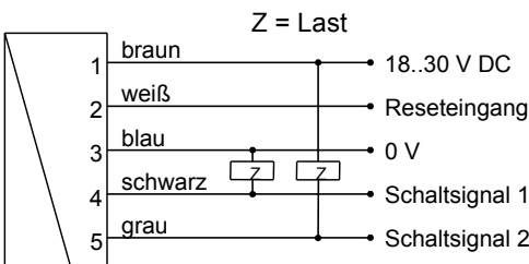
Anschlussbeispiel: PNP NPN
