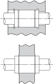
Abb.1 Sicherungsring
