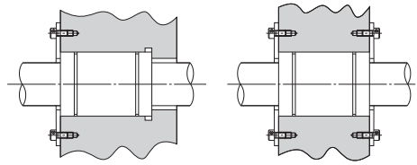
Abb.2 Sicherungsplatte
