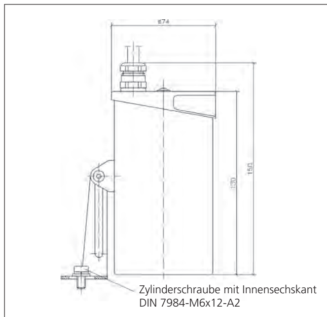
Abmessungen
